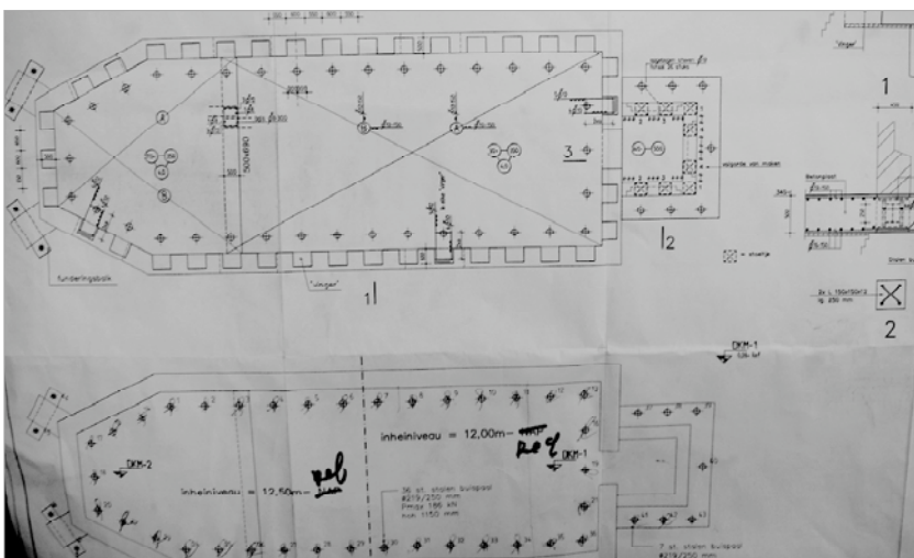
Plaatsing en inheischema van de buispalen.
